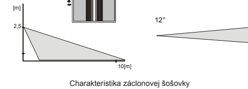
Charakteristika záclonovej šošovky
