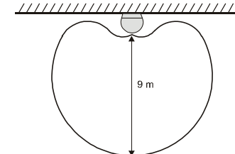
Záběrová charakteristika detektoru rozbití skla
