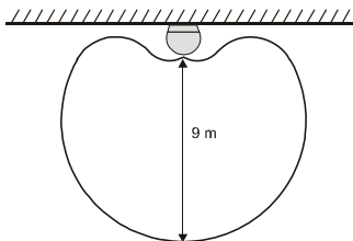
Záberová charakteristika detektora rozbitia skla.
