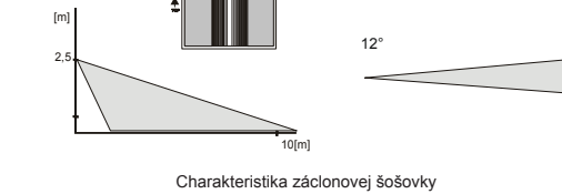
Charakteristika záclonovej šošovky
