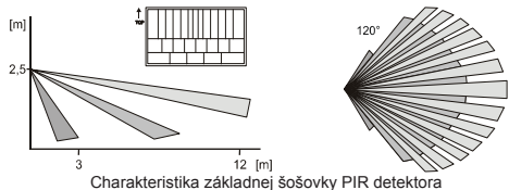
Charakteristika základnej šošovky PIR detektora
