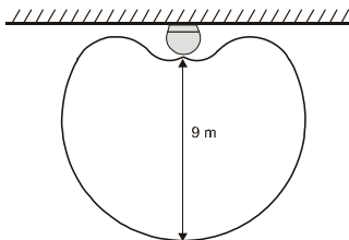
Záberová charakteristika detektora rozbitia skla.
