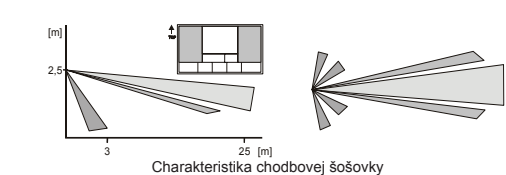
Charakteristika chodbovej šošovky
