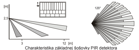
Charakteristika základnej šošovky PIR detektora
