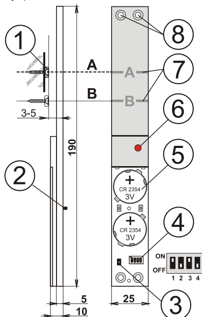
Obrázek: 1. magnet; 2. zadní sabotážní kontakty; 3. sabotážní kontakt krytu; 4. konfigurační přepínače; 5. baterie; 6. signálka LED; 7. detekční značky; 8. montážní otvory
