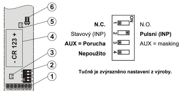
Obrázek 2: Rádiový vysílač: 1 – svorkovnice, 2 – DIP switch pro nastavení chování (z výroby nastaveno – Funkce DIP přepínačů jsou uvedeny v obrázku), 3 – povolení externího ochranného kontaktu, 4 – Držák baterie, 5 – povolení externí antény, 6 – konektor pro připojení externí antény
