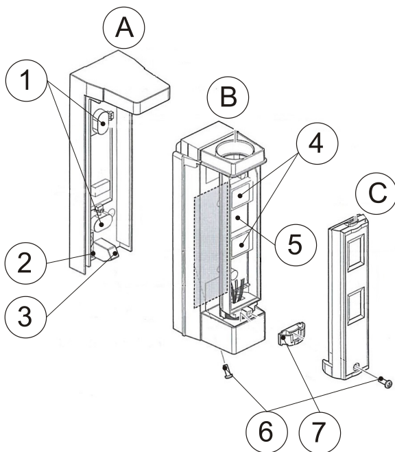
Obrázek 1: Sestava detektoru: A – montážní podložka detektoru, B – základna detektoru s elektronikou, C – čelní kryt detektoru včetně čocek, 1 – otvory pro připevnění detektoru, 2 – trhací část ochranného kontaktu, 3 – dosedací plocha pro kompletaci detektoru se závitem pro stažení šroubem, 4 – čocky detektoru, 5 – DIP switch pro nastavení chování, 6 – aretační šroubky pro kompletaci, 7 – výsuvný fixační třmen
