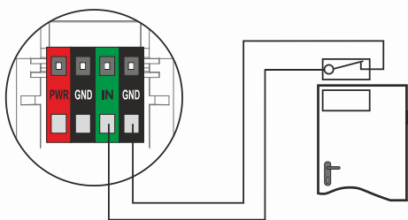
Obr. č. 5: připojení detektoru otevření dveří
