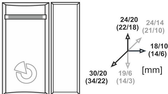
Obrázek 2: vzdálenosti pro aktivaci /deaktivaci detektoru montovaném na nemagnetickém (magnetickém) podkladu
