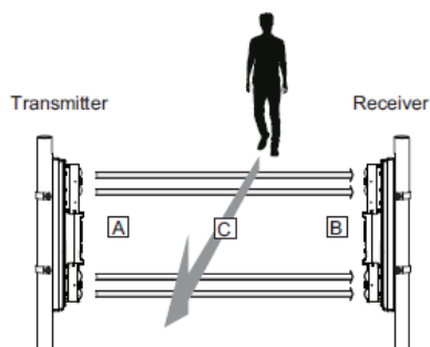
Obr. 8: Provedení testu funkce závory
