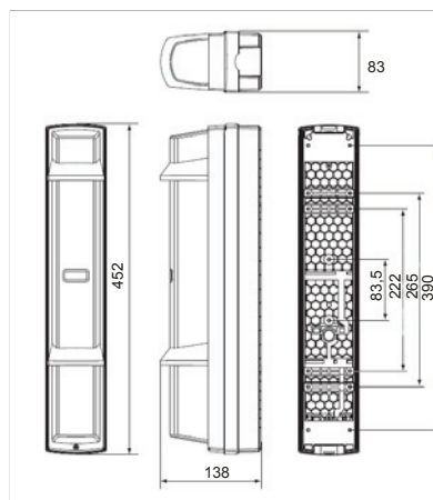
Obr. 10: Rozměry jednotek
