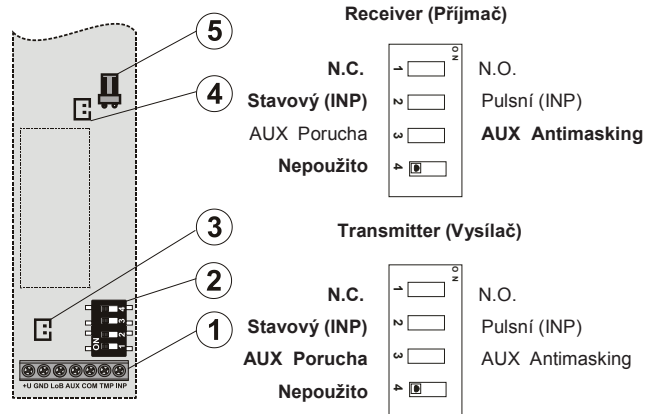
Obr. 3: JA-150TX-V4 Rádiový vysílač (shodné pro vysílač i přijímač jednotku): 1 – svorkovnice, 2 – DIP switch pro nastavení chování (z výroby nastaveno – funkce DIP přepínačů jsou uvedeny v obrázku), 3 – konektor externího ochranného kontaktu, 4 – propojka pro povolení externí antény, 5 – konektor pro připojení externí antény
