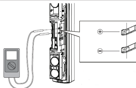
Obr. 5: Seřízení voltmetrem
