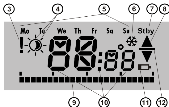
Obrázek 3: 3 – Vstup do vnitřního nastavení ze SW F-Link/Ztráta komunikace; 4 – Symboly komfortní ☀ a ekonomické 🌙 teploty; 5 – Dny v týdnu; 6 – Aktivováno topení při blokování termostatu; 7 – Aktivován režim Vypnuto; 8 – Topení, blikání ▲ – termostat blokován např. otevřeným oknem; 9 – Zobrazení topných časů v ose; 10 – Symboly pro zobrazení teploty, času a textu; 11 – Vybité baterie; 12 – Zobrazení požadované teploty
