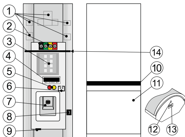
Obrázek 1: 1 – vylamovací otvory pro kabeláž; 2 – svorky sběrnice; 3 – MW senzor; 4 – sériové číslo; 5 – signálky pro indikaci stavů; 6 – konektor pro připojení sabotážního spínače kloubového držáku JA-191PL; 7 – PIR senzor; 8 – sabotážní spínač; 9 – západka elektroniky; 10 – světlovod; 11 – čočka PIR detektoru; 12 – otvor pro aretační šroub; 13 – západka krytu; 14 – přepážka pro ochranu MW senzoru od vodičů
