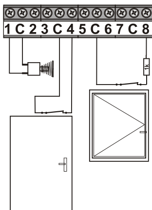
Obrázek: Příklad zapojení přidavného ochranného kontaktu krytu (1-C); rozpínací smyčky (C-4); jednoduše vyvažované smyčky (C-8)
