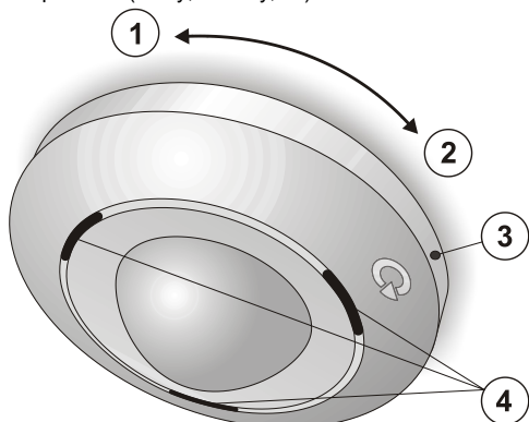
Obrázek 1.: 1 – Směr pro uvolnění detektoru; 2 – Směr pro upevnění (aretační) detektoru; 3 – otvor pro aretační šroubek; 4 – indikační signálky
