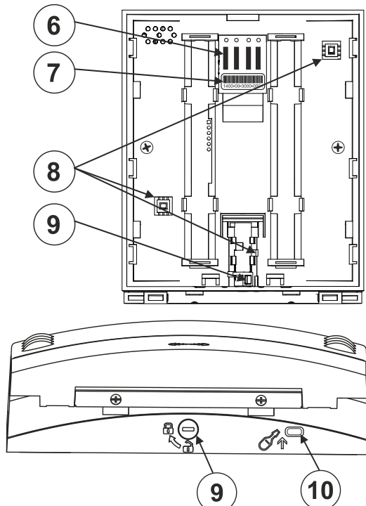
Obr. č. 2: 6 – kontaktní plošky svorkovnice sběrnice; 7 – sériové číslo; 8 – sabotážní kontakty; 9 – aretační mechanismus; 10 – západka
