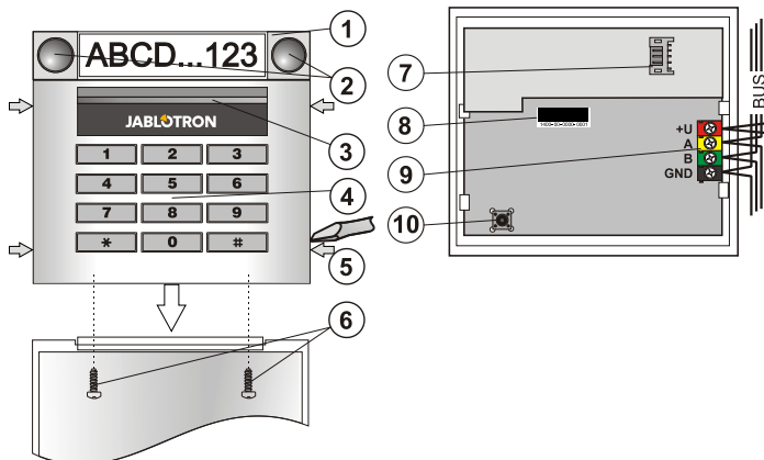
obrázek č. 1: 1 – ovládací segment; 2 – tlačítka segmentu; 3 – prosvětlené aktivizační tlačítko; 4 – přístupový modul se čtečkou RFID; 5 – západky pro otevření modulu; 6 – šrouby krytu;
