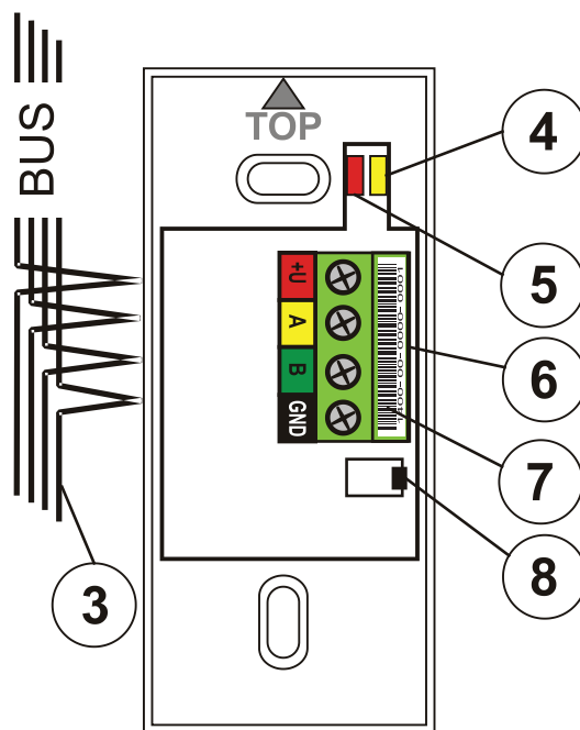
obrázek: 3 – kabel sběrnice; 4 – žlutá signálka porucha; 5 – červená signálka aktivace; 6 – svorky sběrnice; 7 – sériové číslo; 8 – sabotážní spínač
