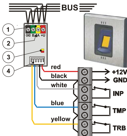
Obrázek: 1 – svorky sběrnice; 2 – sériové číslo; 3 – žlutá signálka indikuje poruchu / nenaucenou periferii, červená signálka indikuje bliknutím aktivaci jakéhokoliv vstupu; 4 – výstupní vodiče viz tabulka:
