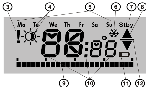
Obrázek 3: 3 – Vstup do vnitřního nastavení ze SW F-Link/ Ztráta komunikace; 4 – Symboly komfortní ☼ a ekonomické ⬤ teploty; 5 – Dny v týdnu; 6 – Aktivováno topení při blokování termostatu; 7 – Aktivován režim Vypnuto; 8 – Topení, blikání ▲ – termostat blokován např. otevřeným oknem; 9 – Zobrazení topných časů v ose; 10 – Symboly pro zobrazení teploty, času a textu; 11 – Nepoužito; 12 – Zobrazení požadované teploty
