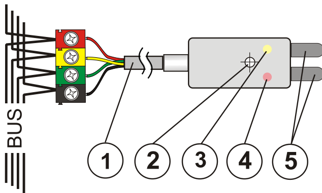
obrázek: 1 – propojení na sběrnici; 2 – montážní otvor Ø 3,1 mm; 3 – žlutá signálka porucha; 4 – červená signálka aktivace; 5 – detekční elektrody (signálky 3 a 4 jsou zality v hmotě detektoru)
